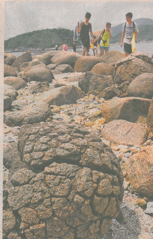
▲石英二長岩的外貌有如菠蘿包面上的裂紋，是地殼內岩漿湧入火山四周裂縫後冷卻形成的岩石。受海水侵蝕及冷縮熱脹影響，表層與內部產生裂縫逐漸層層剝落，又稱為頁狀剝落。
